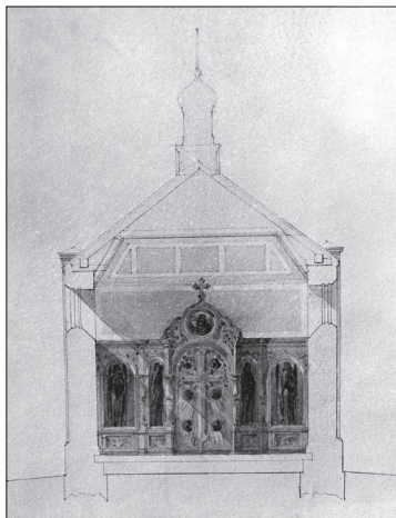
Проект расширения часовни. Разрез. Вид иконостаса. 1858 г.
